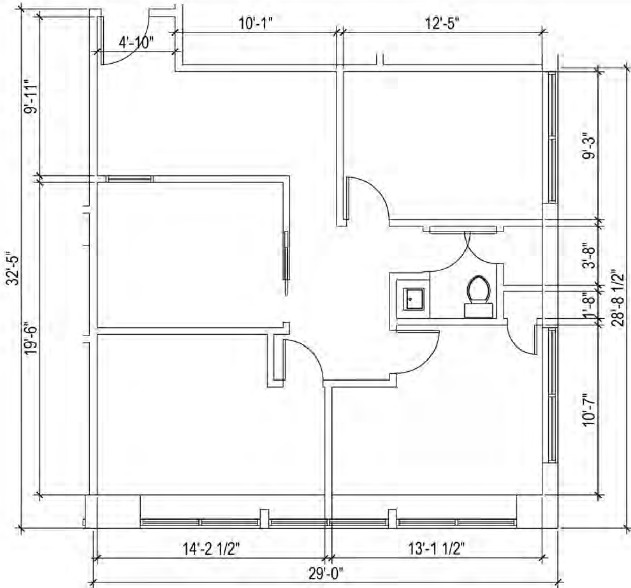
1 SUITE 221 PLAN - 855 S.F.
